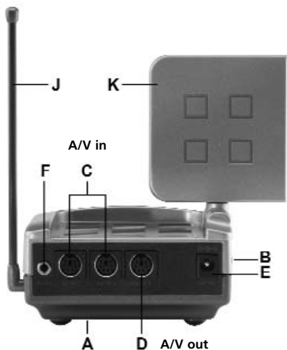
Abbildung 3 A/V SENDER
